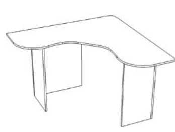
Стол угловой правый 1500 x 770 x 1200
