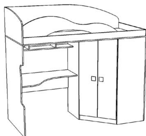
Кровать 2-этаж + шкаф 2032 x 1870 x 852
